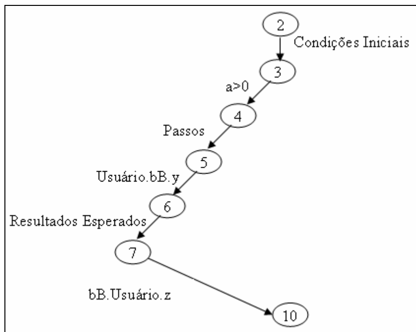
Figura 3.5 - Construção do LTS derivado do diagrama de seqüência da Figura 2.7 – Fluxo alternativo 1
