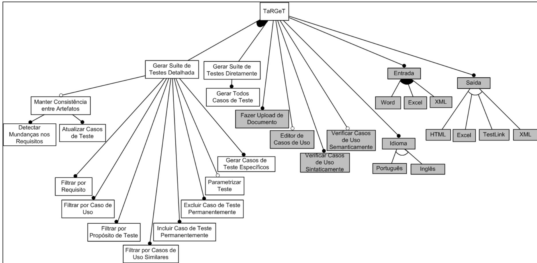
Figura 26 - Modelo de features de TaRGeT refinado
