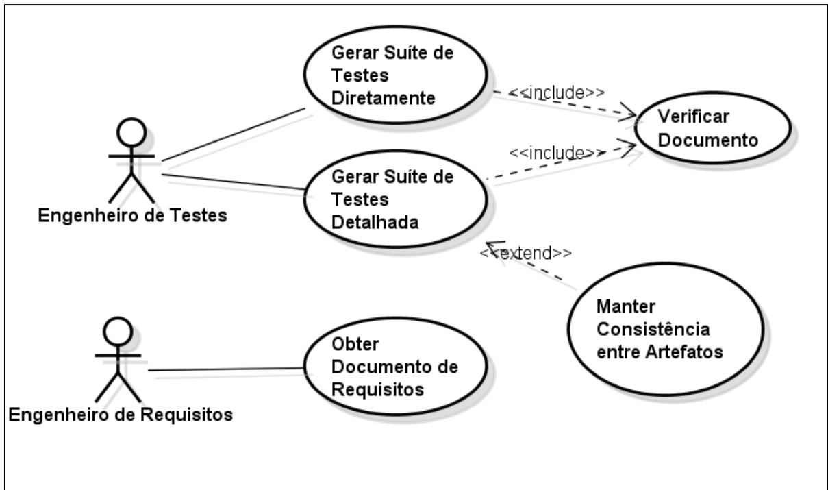
Figura 27 - Diagrama de casos de uso de TaRGeT
